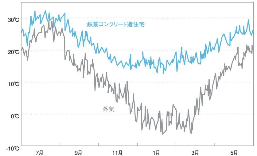
■鉄筋コンクリート造住宅と外気の1年間の変化
