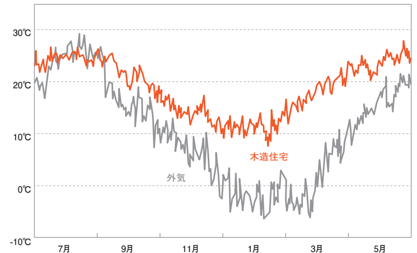
■木造住宅と外気の1年間の変化
